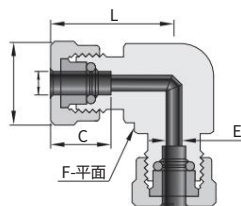
彎頭
