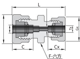
縮徑直通
